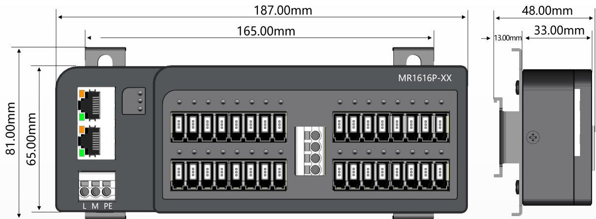
图2 尺寸 187 *81 (W/H, mm)
