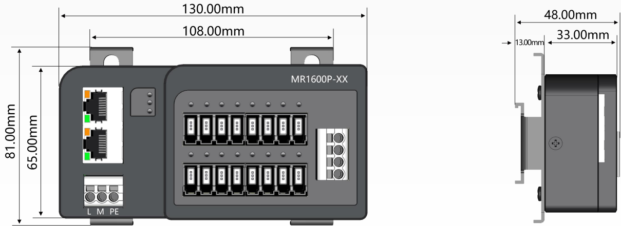
图1 尺寸 130*81 (W/H, mm)
