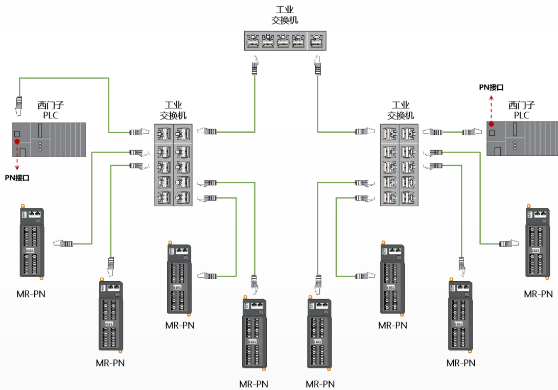
图 6-3 PROFINET 树形网络拓扑结构
