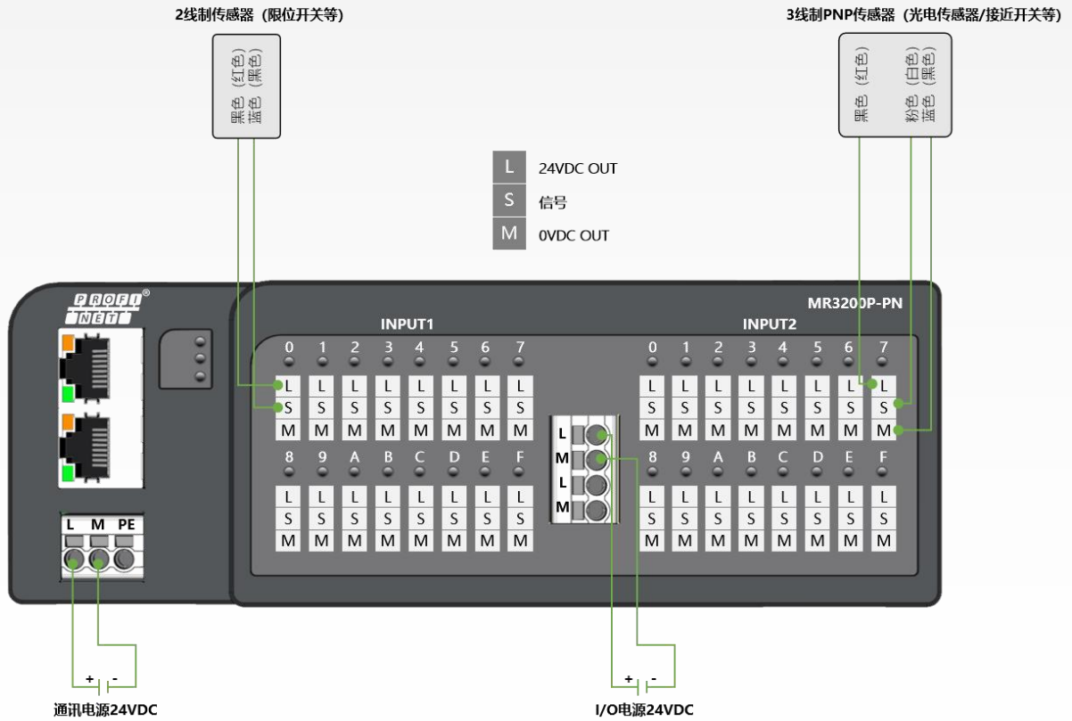
32 点输入 PNP
