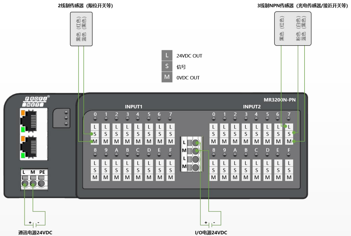
32 点输入 NPN
