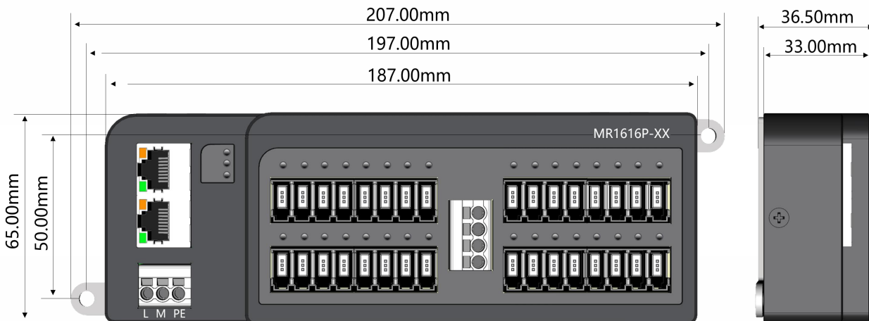
图 4 尺寸 1--207 *65 (W/H, mm)
