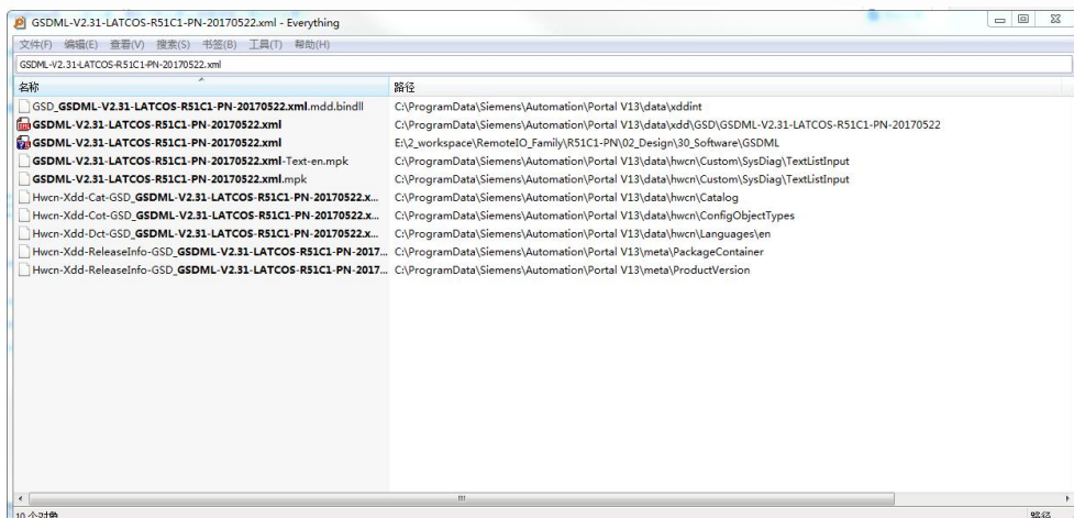
图 7-5 Everything 窗口
